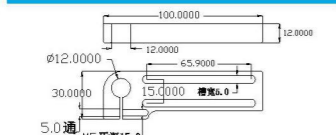
固定支架 JD-A12
