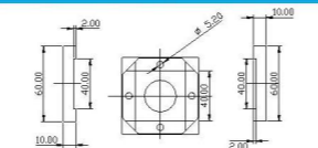
铝条固定支架 JD40-40
