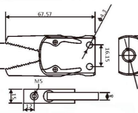
迷你夹具 C
