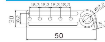
双槽迷你夹具支架 JD20E-097
