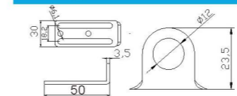
双槽金具L型支架 JD20E-105
