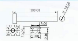
气动手指固定支架 JD-M10
