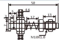
JD07-1050 小头金具
