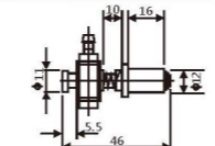
VFIL-S-10-P12 铝大头金具
