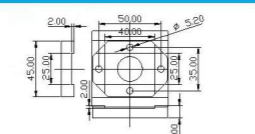
铝条固定支架 JD25-40
