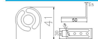
双槽迷你支架L型支架 JD20E-101
