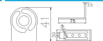
双槽迷你支架L型支架 JD20E-102
