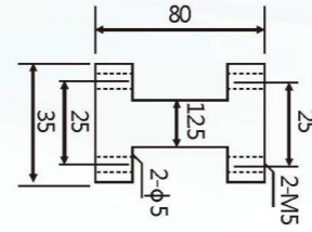
小夹具连接工字架80mm
