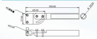
万向可调支架 JD12-H20
