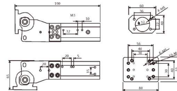
产品型号: JDCZ-3240 重量: 1.2kg 可搬重量: 5kg
