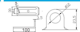
双槽金具L型支架 JD20E-107
