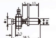
VFIL-SS-5-P8 铝小头金具
