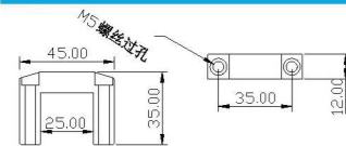
铝条固定支架 JD-25
