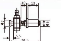
VFIL-SS-10-P8 铝小头金具
