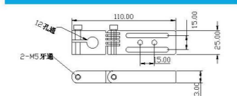
角度调整链接件 JD-D12
