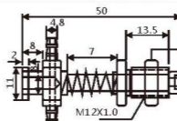
JD11-1250 大头金具
