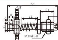
JD11-1055 大头金具
