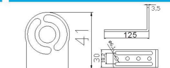
双槽迷你支架L型支架 JD20E-104
