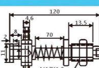
JD11-12120 大头金具
