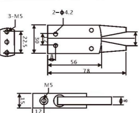
迷你夹具 B
