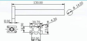
气动手指固定支架 JD-M16
