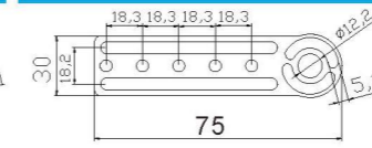
双槽迷你夹具支架 JD20E-098
