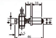
VFIL-S-5-P12 铝大头金具
