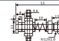
JD11-1253 大头金具
