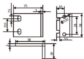
小夹具连接L块75mm
