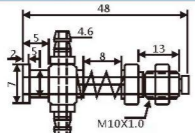
JD07-1048 小头金具
