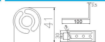
双槽迷你支架L型支架 JD20E-103
