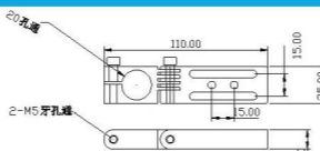
角度调整链接件 JD-D20
