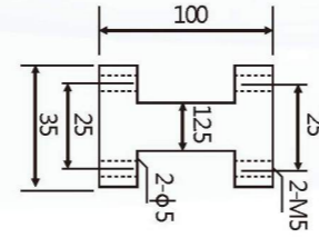
小夹具连接工字架100mm
