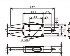
迷你夹具EX-20
