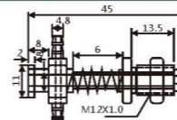
JD11-1245 大头金具
