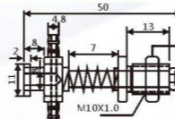
JD11-1050 大头金具
