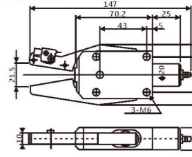
迷你夹具EX-20-C
