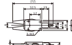
迷你夹具EM1-08
