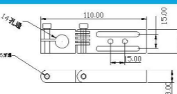
角度调整链接件 JD-D14
