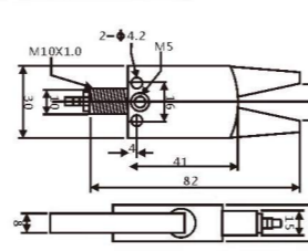
迷你夹具 D
