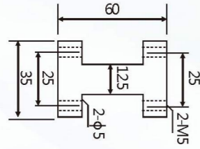
小夹具连接工字架60mm
