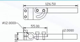
万向可调支架 JD12-H12
