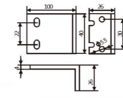
大夹具连接L块100mm
