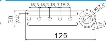
双槽迷你夹具支架 JD20E-100
