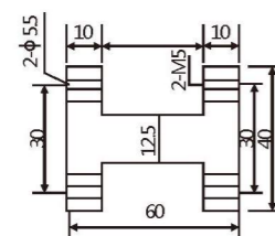
大夹具连接工字架60mm
