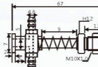
VFIL-SS-30 铝小头金具
