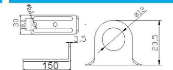
双槽金具L型支架 JD20E-108
