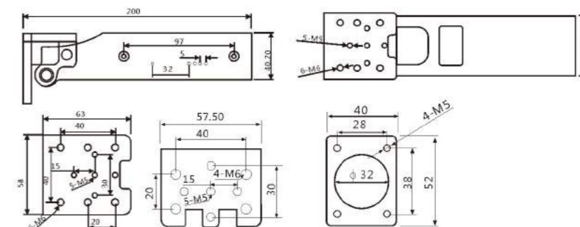
产品型号: JDCH-3240DL 重量: 1kg 可搬重量: 5kg
