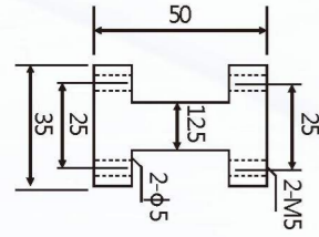
小夹具连接工字架50mm
