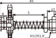
VFIL-S-5 铝大头金具
