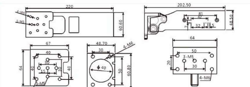
产品型号: JDCH-4040DL 安装孔: 30x50mm 重量: 1.3kg 可搬重量: 10kg
