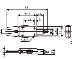
迷你夹具EM-12
