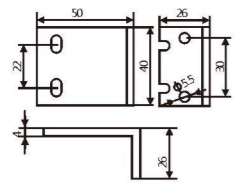
大夹具连接L块50mm
