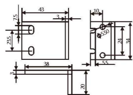
小夹具连接L块43mm
