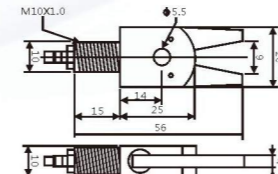
迷你夹具 E
