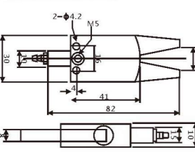
迷你夹具 A
