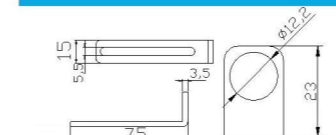
单槽金具L型支架 JD20E-109
