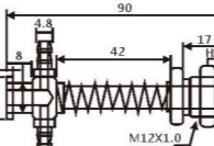
VFIL-S-40 铝大头金具
