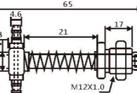
VFIL-S-20 铝大头金具
