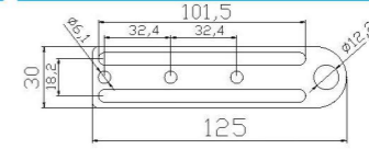
金具固定板G JD20E-095
