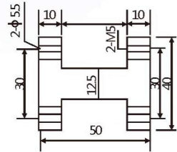
大夹具连接工字架50mm
