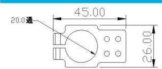
管道夹具垫片
