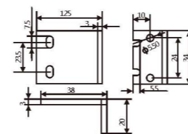
小夹具连接L块125mm
