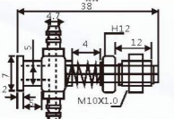
VFIL-SS-5 铝小头金具
