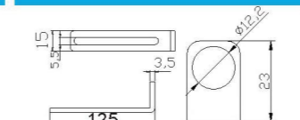
单槽金具L型支架 JD20E-110
