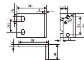
小夹具连接L块100mm
