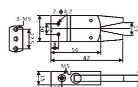
迷你夹具BK
