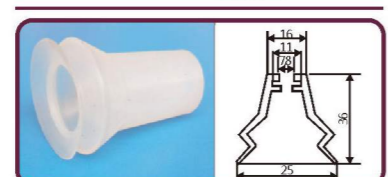
JD2-25 瓶坯吸盘
