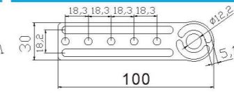
双槽迷你夹具支架 JD20E-099
