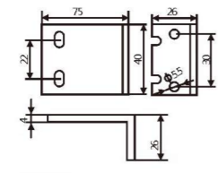
大夹具连接L块75mm
