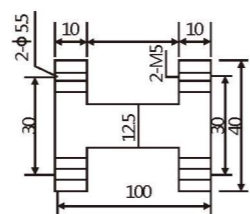
大夹具连接工字架100mm
