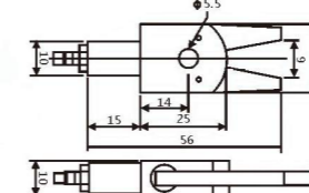
迷你夹具 F
