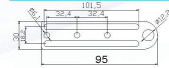
金具固定板E JD20E-093
