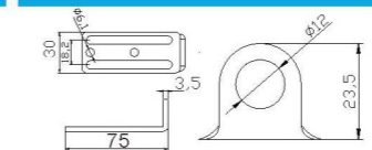
双槽金具L型支架 JD20E-106
