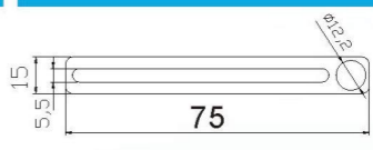
单槽金具平面支架 JD20E-111
