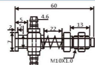
JD07-1060 小头金具
