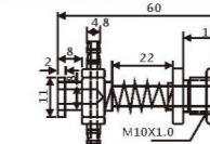
JD11-1060 大头金具
