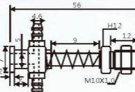
VFIL-SS-20 铝小头金具
