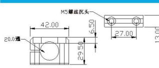
固定支架 JD-Φ20
