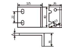
大夹具连接L块125mm
