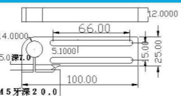
固定支架 JD-A14
