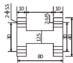
大夹具连接工字架80mm
