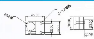
铝条固定支架 JD25-Φ20
