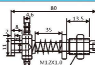
JD11-1280A 大头金具
