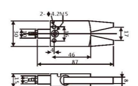
迷你夹具AK
