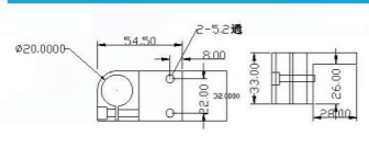
铝条固定支架 JD40-Φ20
