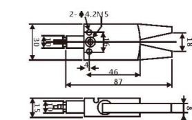
迷你夹具AH (带磁)
