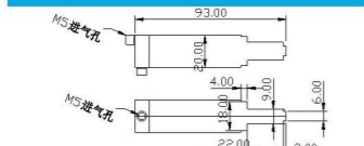
顶出节吸金具 JD20-H90
