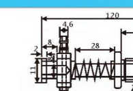
JD11-12120B 大头金具加长牙
