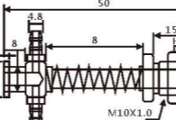
VFIL-S-10A 铝大头金具
