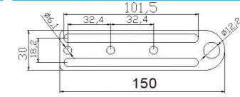
金具固定板H JD20E-096
