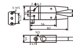
迷你夹具BH (带磁)
