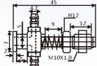
VFIL-SS-10 铝小头金具
