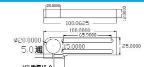
固定支架 JD-A20
