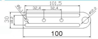
金具固定板F JD20E-094
